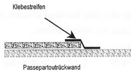
Querschnitt:
